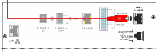
Face arrière du premier afficheur AFFseries-3
