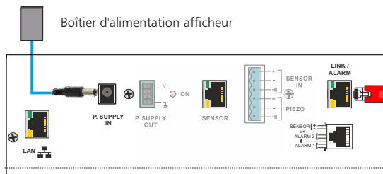
Face arrière du deuxième afficheur AFFseries-3
